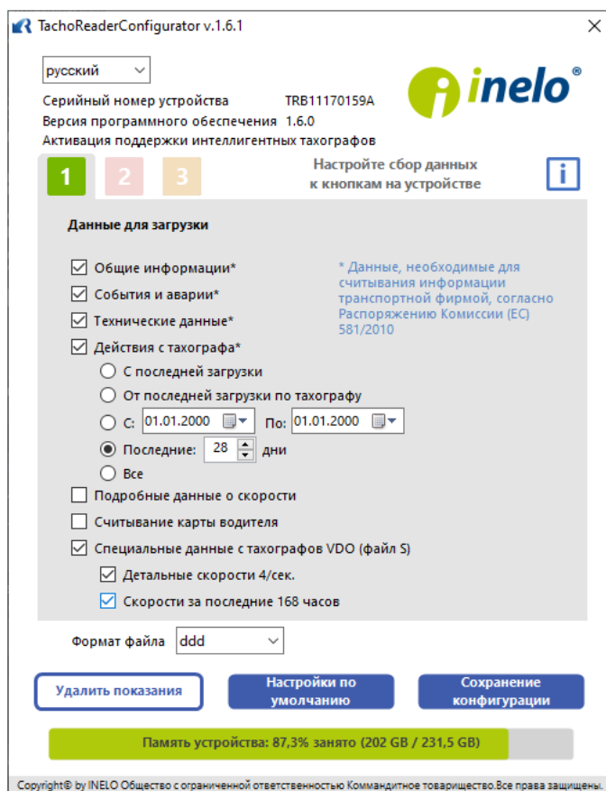
Рис. Окно конфигурации устройства: TachoReader Basic.
