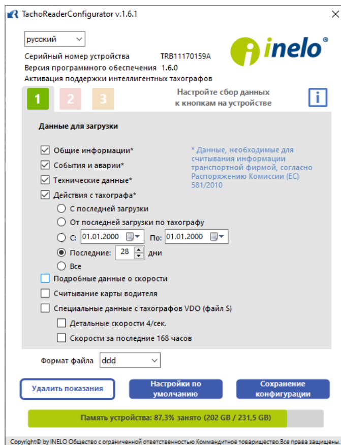
Рис. Окно конфигурации устройства.
